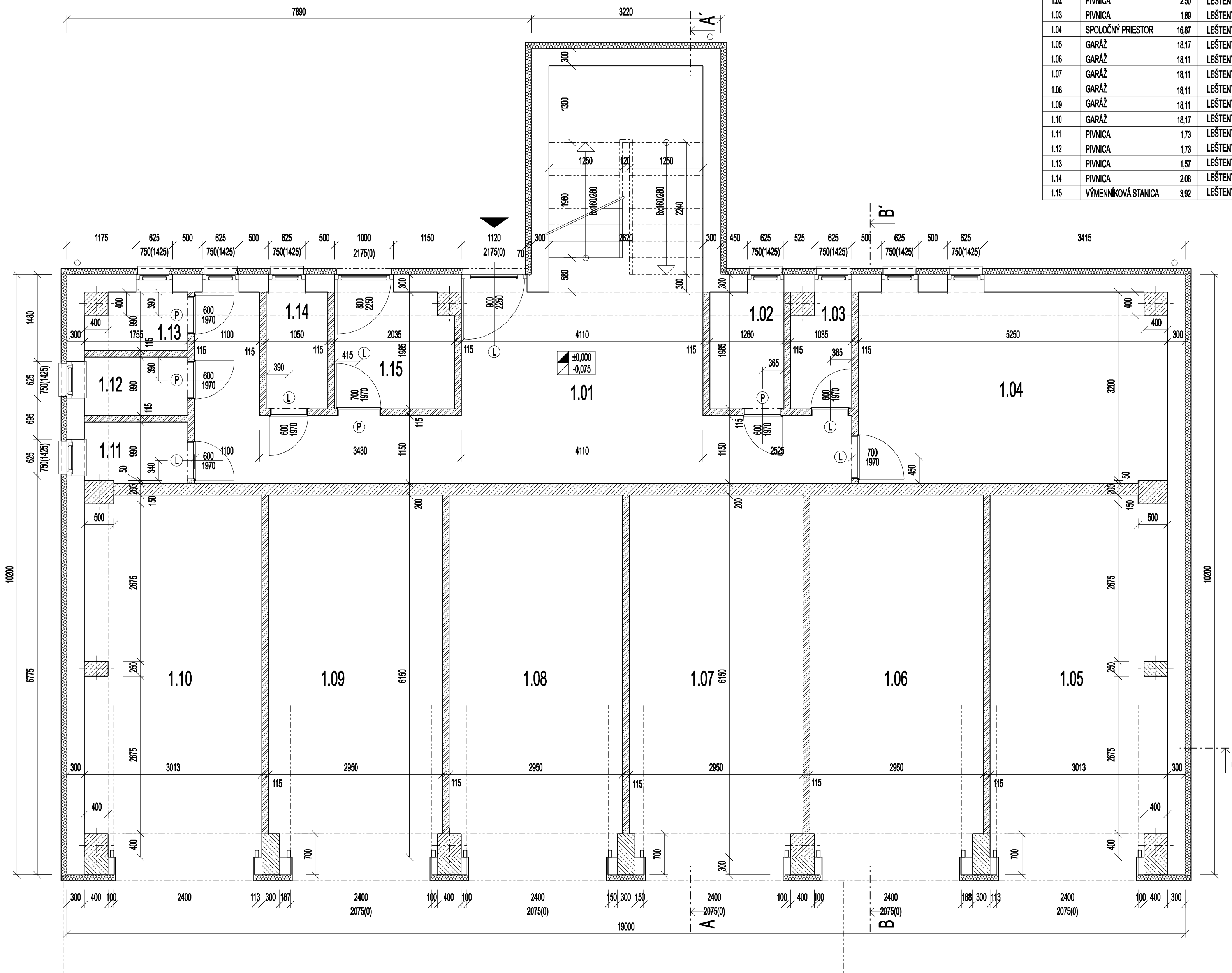
PÔDORYS PRÍZEMIA
